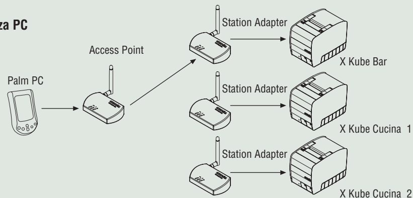
Esempio di configurazione X Kube Wi-Fi
